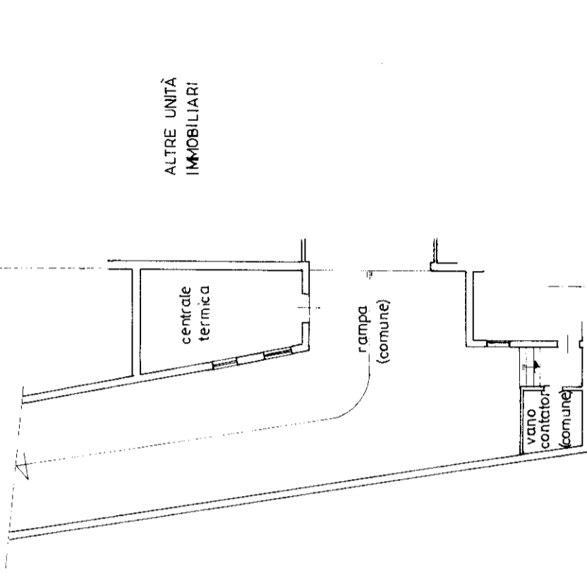
PIANTA PIANO INTERRATO H=3.25 mt.
